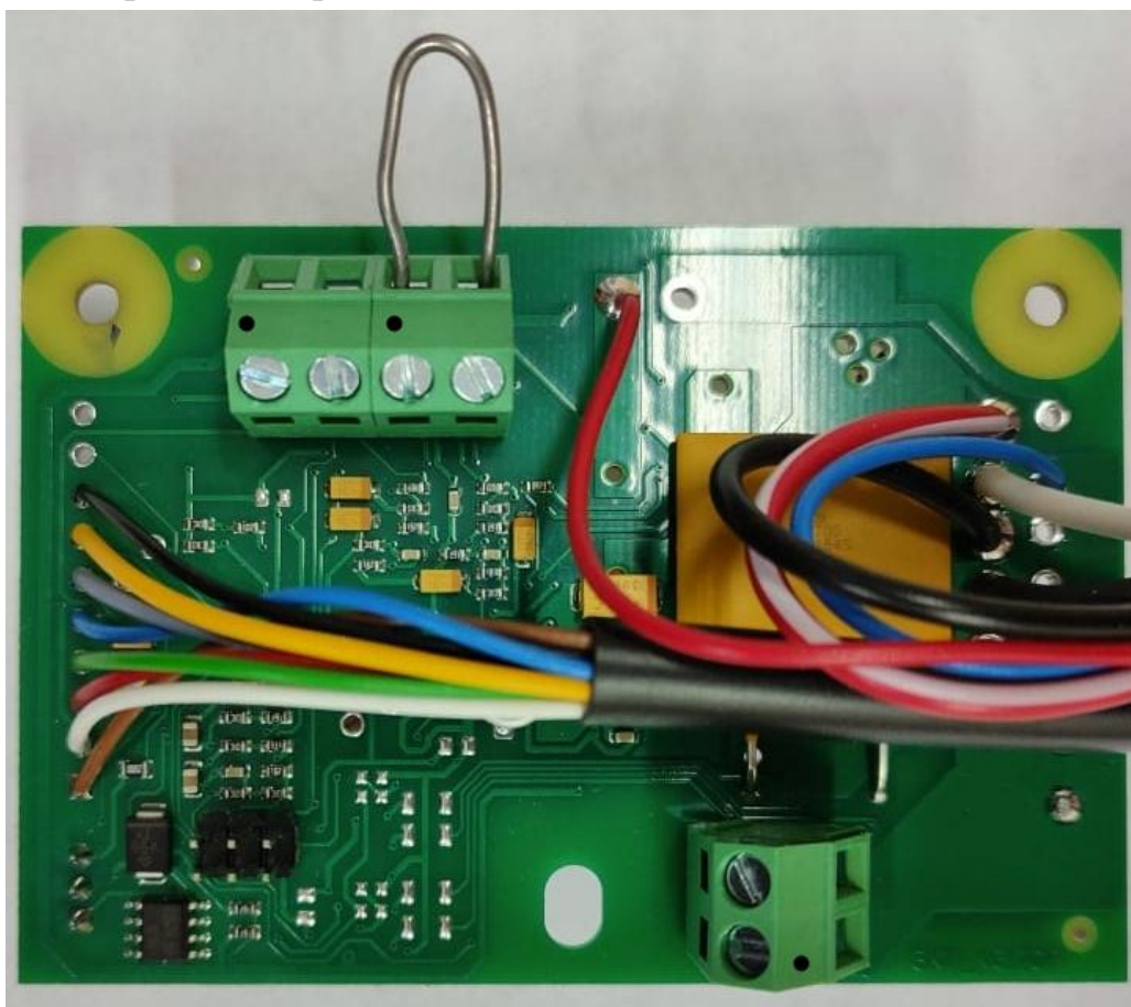
Рис. 8 – Перемычка
