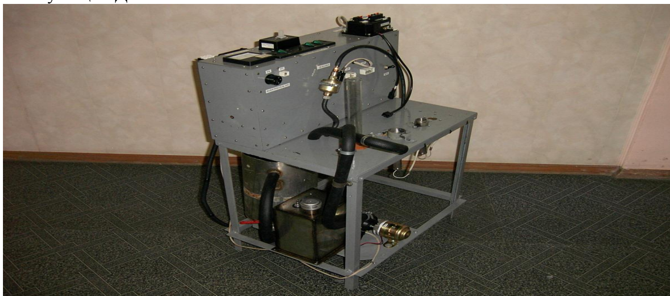
Рис 21- Стенд контроля
