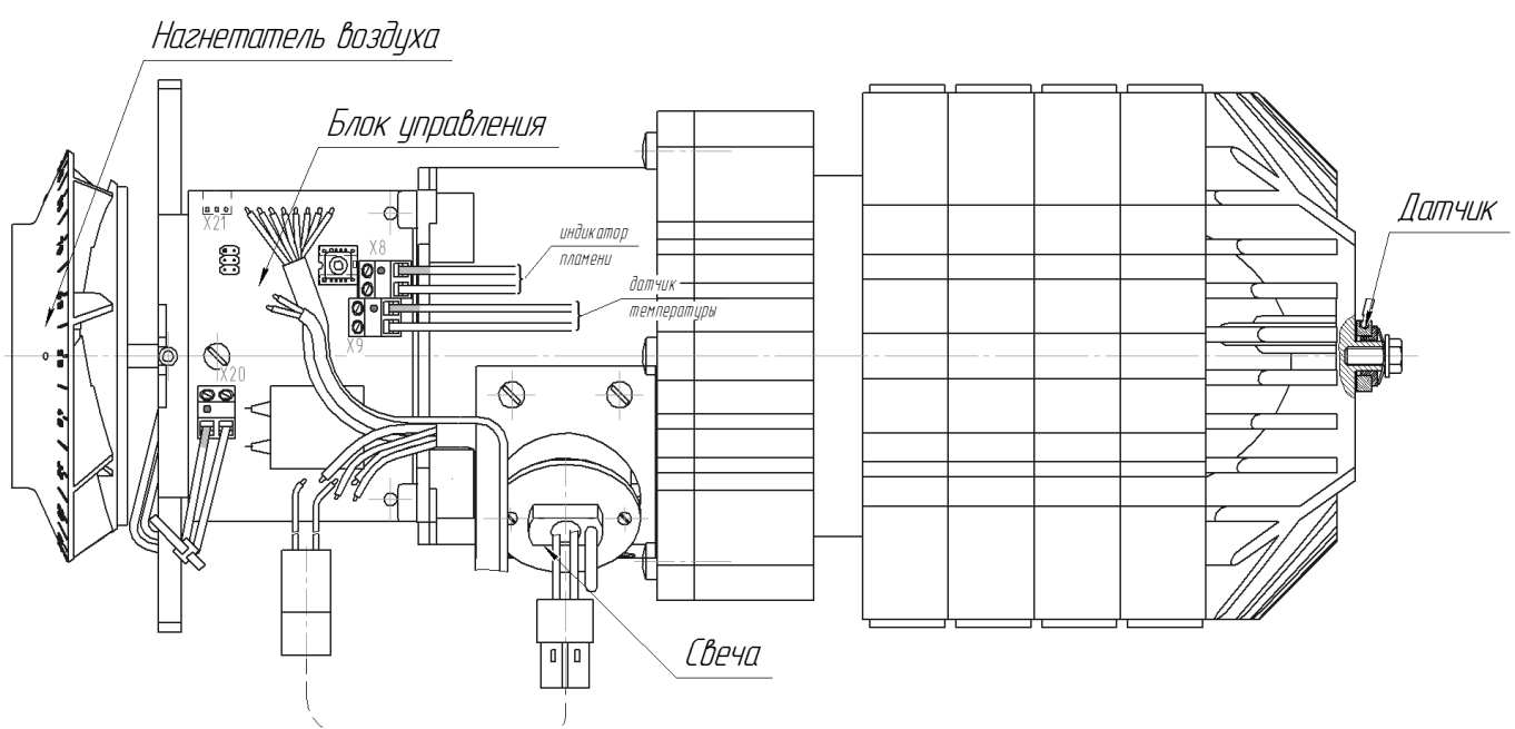
Рис.2 – Нагреватель.
